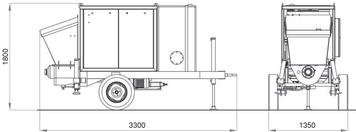
Adroit 007
