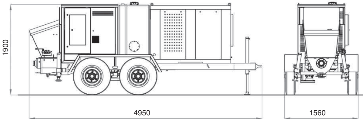
Adroit 007C
